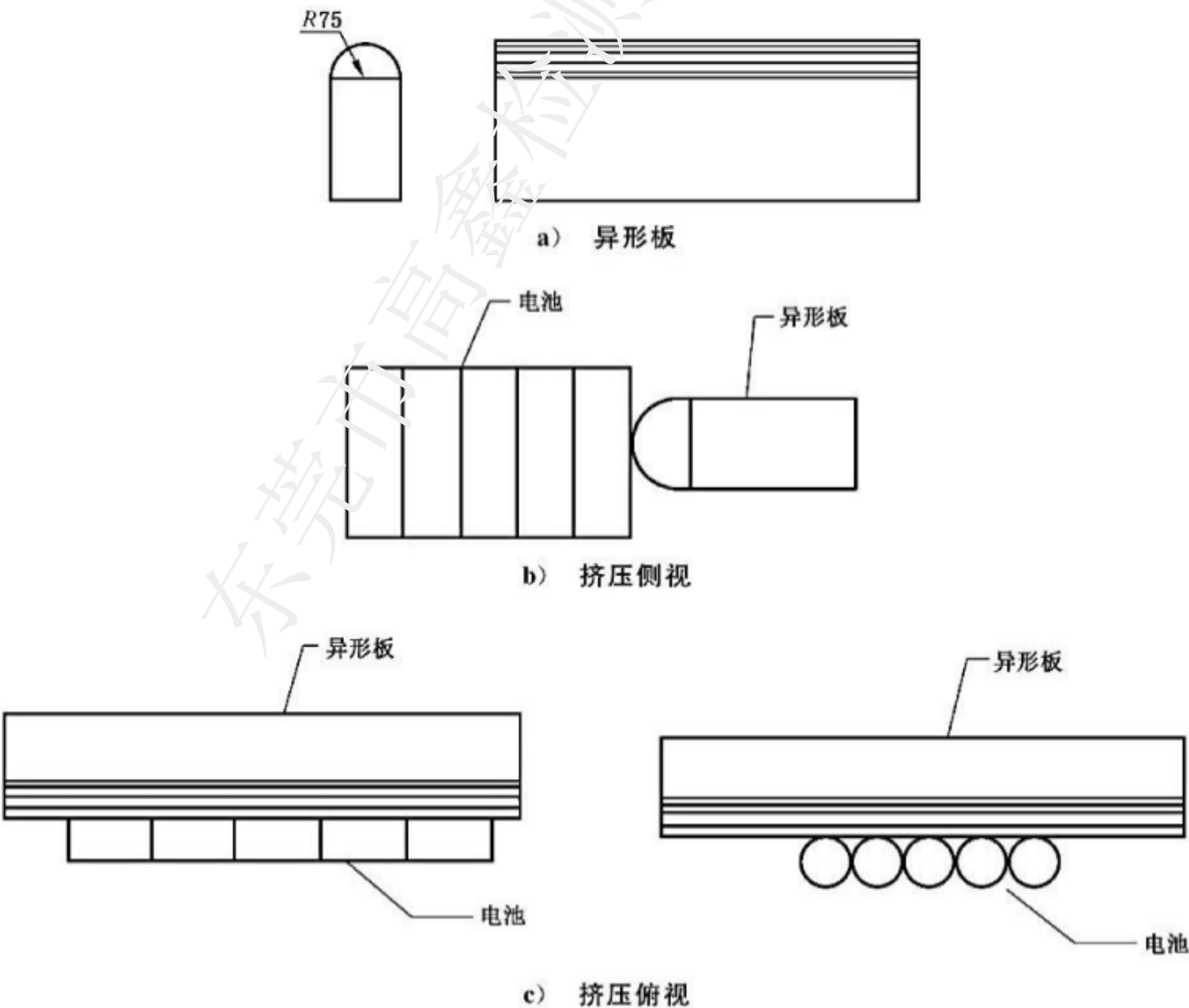
图 1 异形板和挤压示意图
